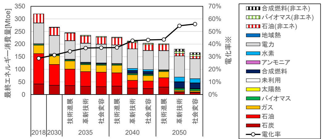
図 2 最終エネルギー消費量と電化率の推移
