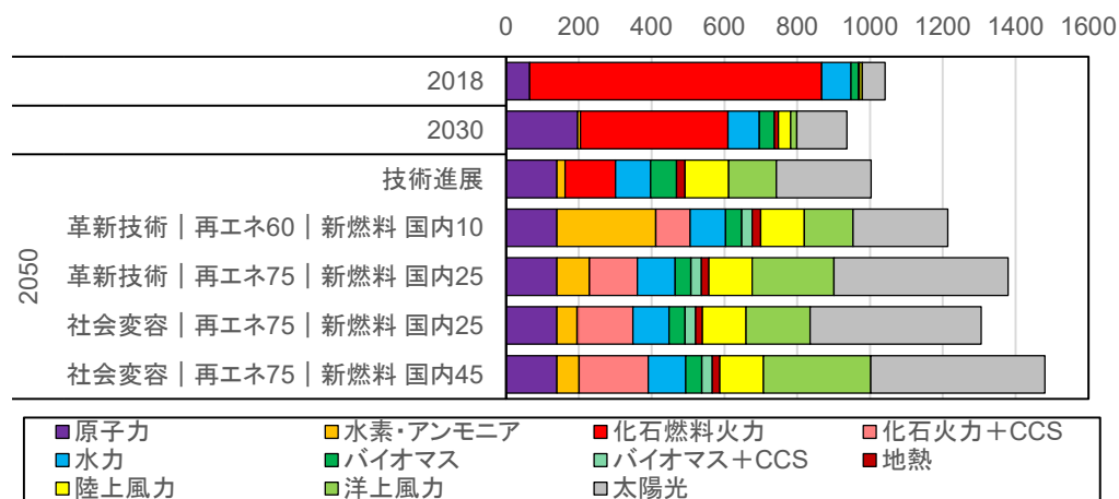
図3 発電電力量とその内訳(単位:10 億 kWh)
